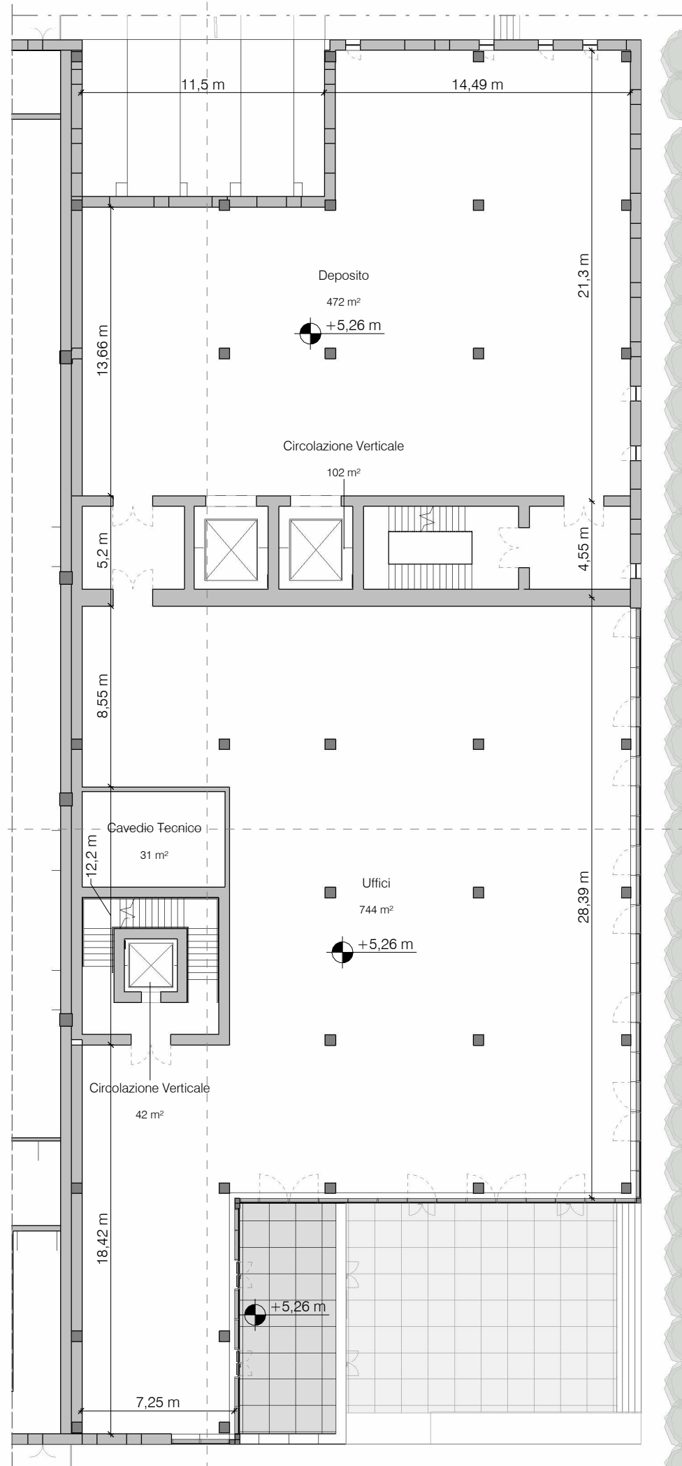
Pianta Livello 1 1:250
