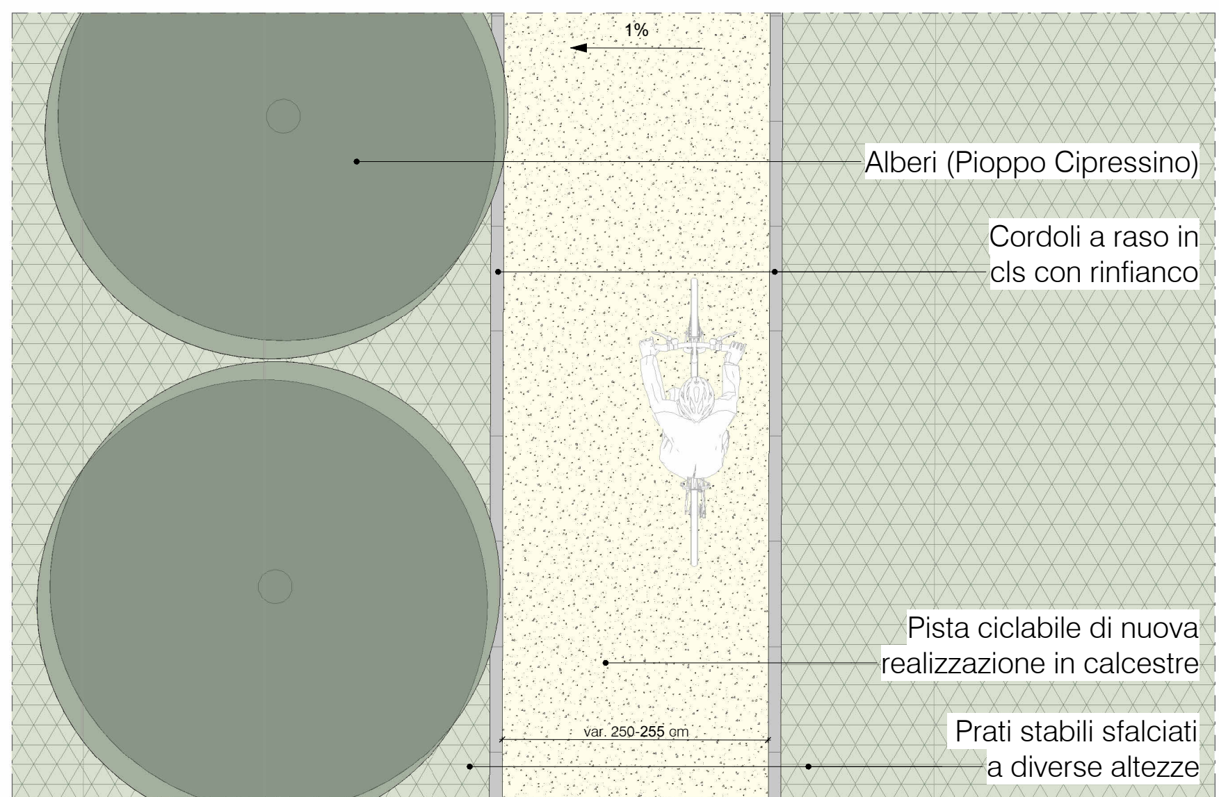
Stralcio pianta pista ciclabile 1: 50
