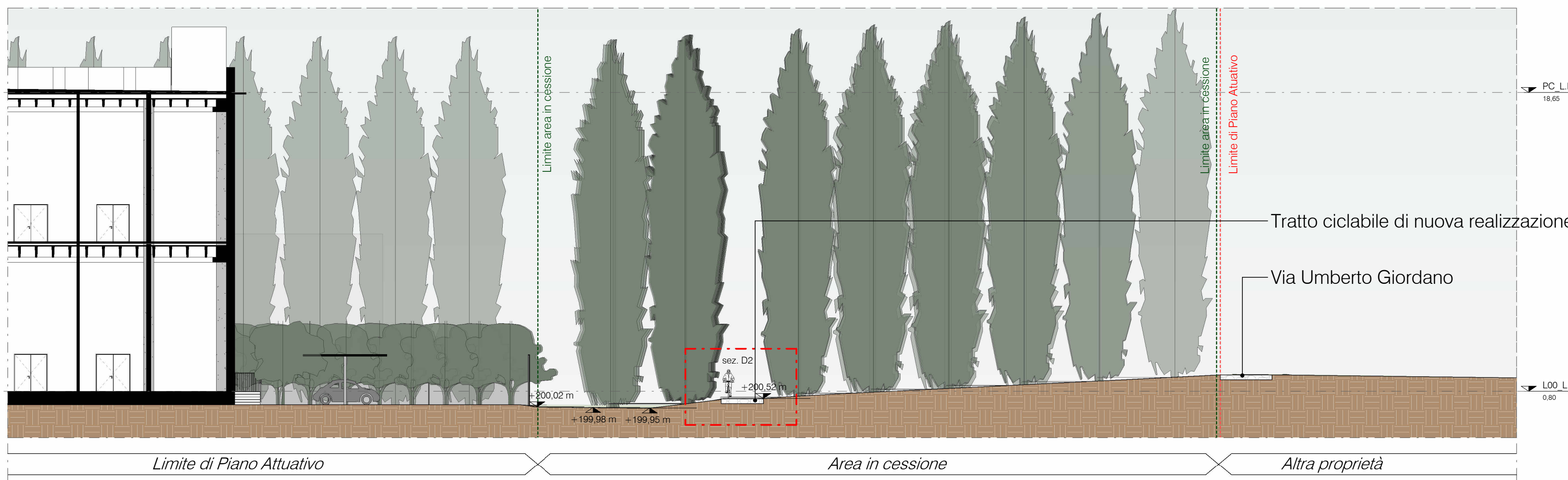
Sezione D1 1: 200
