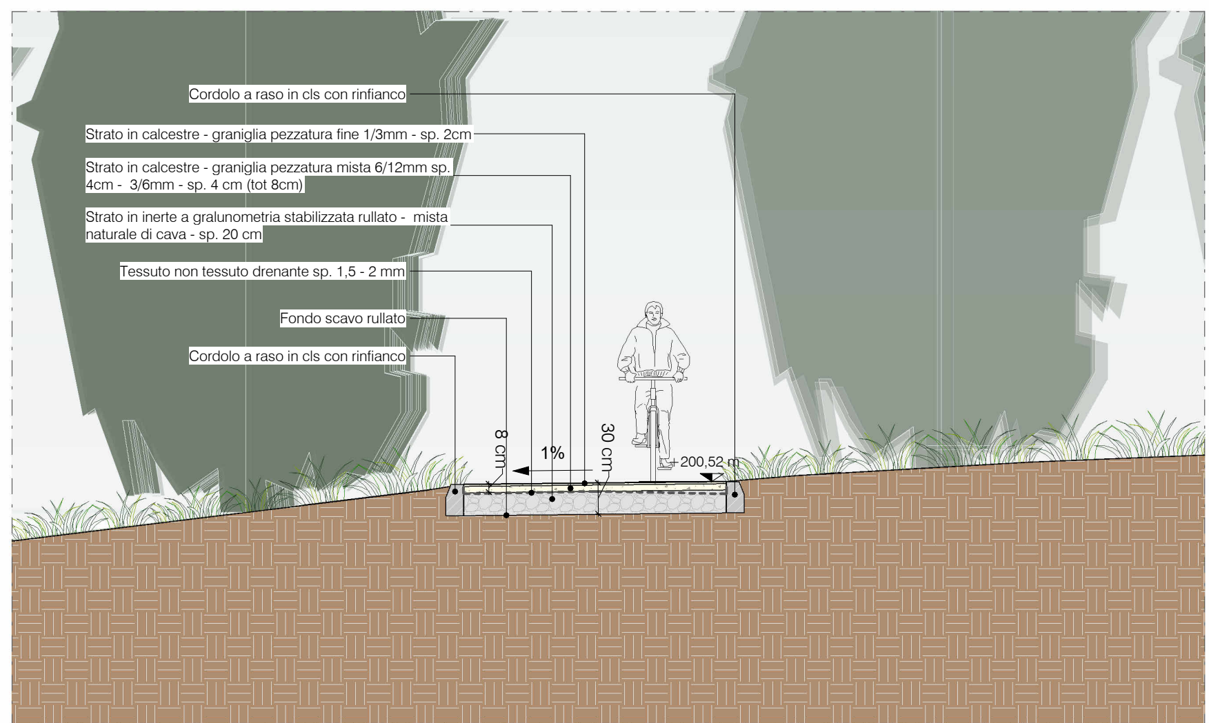
Sezione D2 - Sezione tipo pista ciclabile 1: 50
