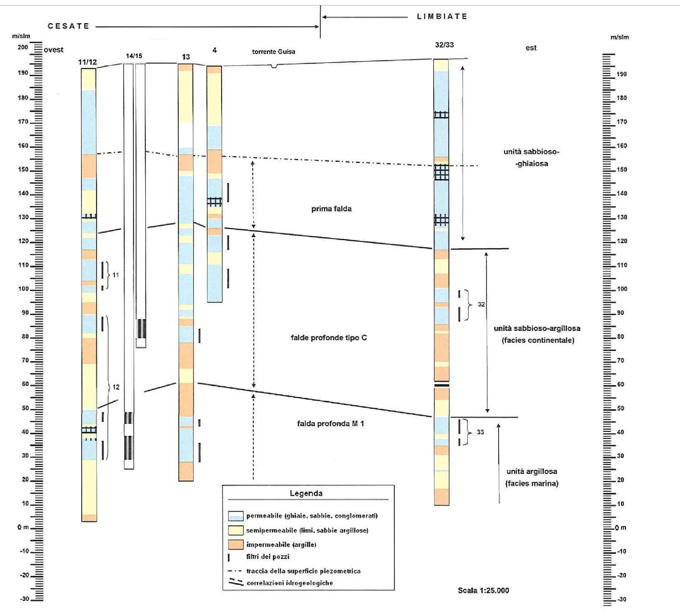
Sezioni idrogeologiche tratte da "Studio per realizzazione nuovo pozzo in comune di Cesate", a cura di CAP Holding Spa - novembre 2008
